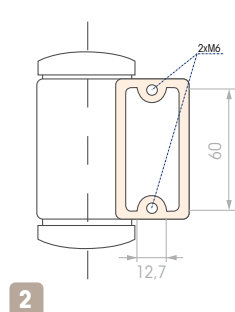
Haltebock direkt verschraubt
