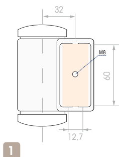
Haltebock über Sechskant verschraubt
